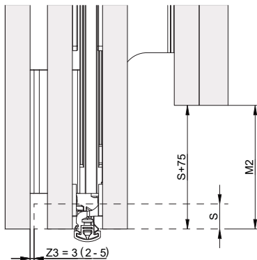
Türe bündig
