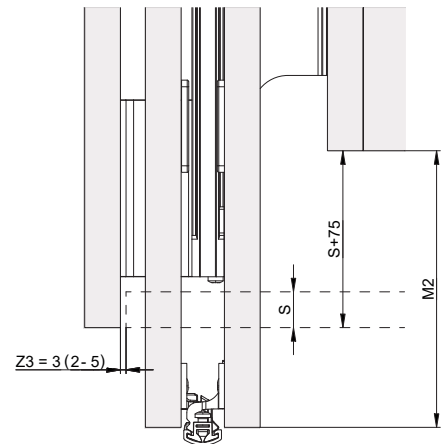
Türe vorstehend
